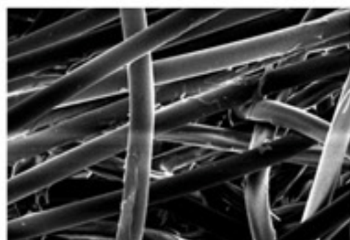
●3M™菌を吸着する除菌用シート表面の顕微鏡写真 (X750)
